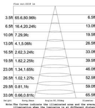
LTL-150W-CW
