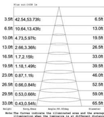
LTL-100W-CW
